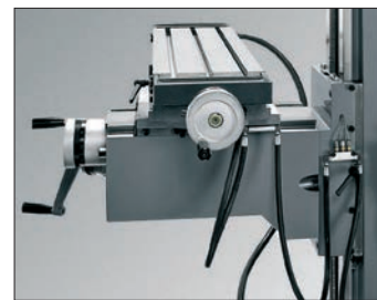
Cod. 40007: Graissage centralisé
