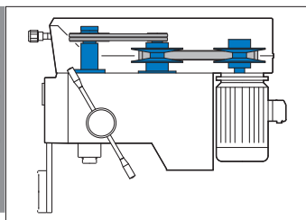
VS: Variateur simple
