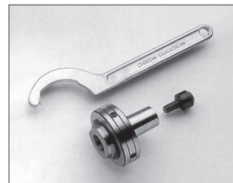
Cod. 39000050/60/70: Cône avec écrou de serrage pour fraises à queue conique (CM1, CM2 ou CM3 sur demande)
