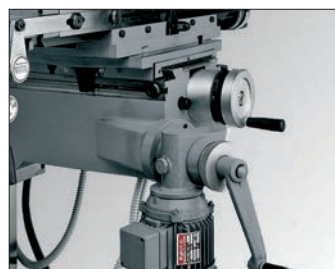
Cod. 40006: Avance rapide verticale de la table
