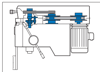
VH: Variateur harnais
