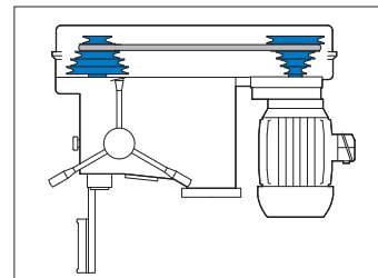
PU (E): Poulies étagées électronique V22E
