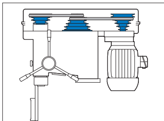
PU: Poulies étagées V30
