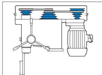
PU: SPoulies étagées électronique V22 - V25 - V25E.
