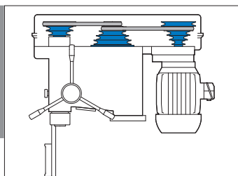
PU: Poulies étagées V22 - V25 - V25E.
