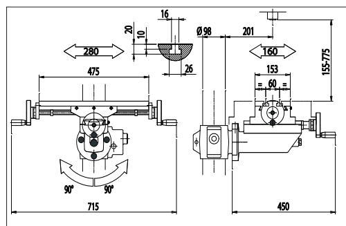
TC: Table Croisée.
