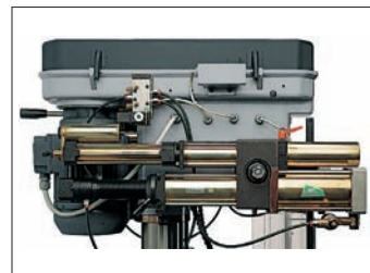
Cod. 30019: Descente hydropneumatique. Course automatique de la broche de 90/105 mm avec retour, rapide. Avance: 5 à 2500 mm/1' Effort de poussée à 6 bar: 400 Kg.
